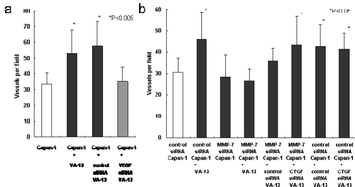
図1 線維芽細胞VA-13由来VEGFはCTGFにより不活性化され、腫瘍内でがん細胞の産生するMMP-7により再活性化される。種々のsiRNAで処理したがん細胞Capan-1と線維芽細胞VA-13をヌードマウス皮下に植え形成された腫瘍の血管密度を2週後に評価した。a. 線維芽細胞VA-13由来VEGFの腫瘍血管密度への影響 b. がん細胞Capan-1由来MMP-7と線維芽細胞VA-13由来CTGFの影響
