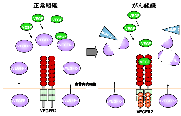
図4 血管内皮細胞周囲におけるVEGF活性制御に関するモデル 正常環境では血管内皮細胞の周囲に産生されるsVEGFR-1の作用によりVEGFは血管内皮細胞にアクセスできない。 がん環境ではMMP-7の作用によりsVEGFR-1が分解されることでVEGFが開放、血管内皮上のレセプターに結合し、血管新生を亢進する。
