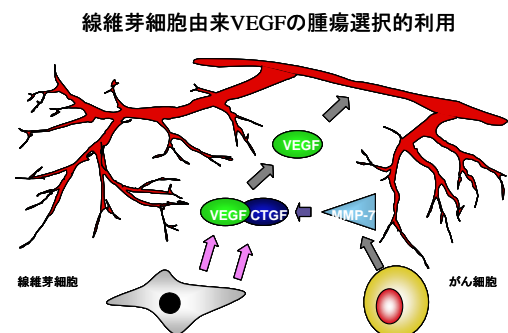
図2 線維芽細胞由来VEGFの活性制御に関するモデル。正常組織では線維芽細胞由来のVEGFはCTGFの作用により不活性化される。がん組織ではがん細胞由来のMMP-7の作用で再活性化され血管新生を亢進する。
