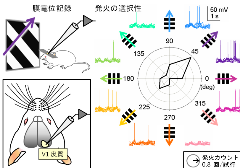
図 1. マウス一次視覚皮質の方向選択性 (左上) 格子刺激の提示と膜電位記録 (左下) 一次視覚 (V1) 皮質の座標 (右) 代表的な V1 ニューロンの膜電位応答と発火の選択性
