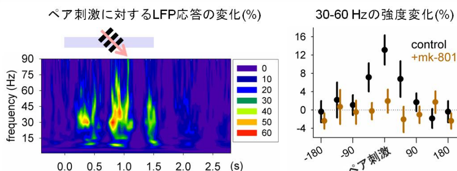
図4. フラッシュとのペアリングによるLFP応答の変化 (左) パワースペクトログラムの比 (ペアリング後/ペアリング前) から得られた各周波数成分のLFP応答強度の変化 (右) 各格子刺激に対するLFP応答のガンマ強度 (30-60 Hz) の変化
