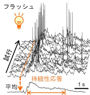
図3. フラッシュに対するV1ニューロンの膜電位応答
