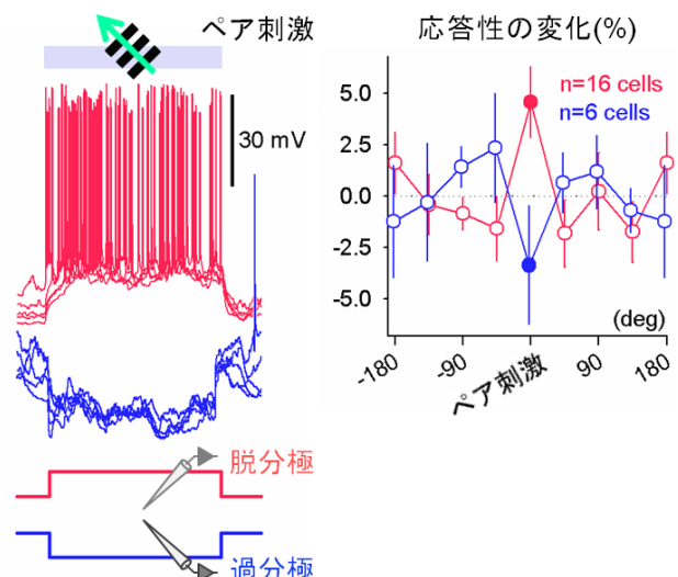
図 2. 電流注入とのペアリングによる発火選択性の変化 (左) 特定の格子刺激 (ペア刺激) 提示時に、脱分極性ないし過分極性の電流を注入する (右) ペアリングによる発火応答の変化 (恣意的な尺度)
