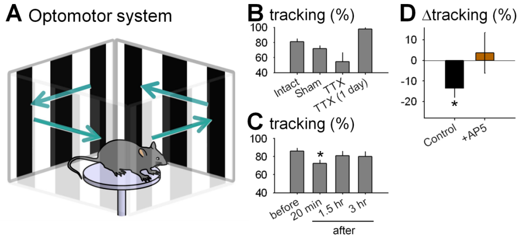
図5. A) オptomotor・システムの模式図。プラットフォームの周囲に格子模様を描いたモニター4台を配置し、マウスをプラットフォーム上に自由行動させる。モニター上の格子模様をさまざまなインターバルで左右いずれかに動かした際の、マウスの追尾行動 (tracking) の有無を検出する。B) V1 への局所的な TTX 処置前、処置直後、一日後の tracking 率 (n=4 mice)。C) フラッシュとのペアリング前および 20 min, 1.5 hr, 3 hr 後の paired 方向への tracking 率 (n=16 mice)。D) V1 への局所的な AP5 処置を施した群および無処置群 (control) における tracking 率の変化 (n=12 mice for AP5)。( * p < 0.05 , paired t -test, vs before)
